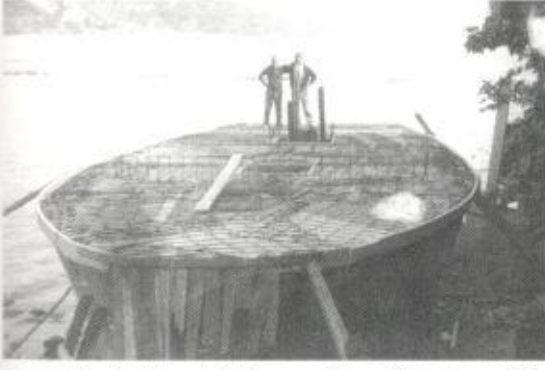
Solda Kapt. Necdet Musaoğlu sağda Nurettin Şairoğlu ile inşa ettikleri beton tekne. (Bu tekne tamamlanmış ve çalışmıştır.)
